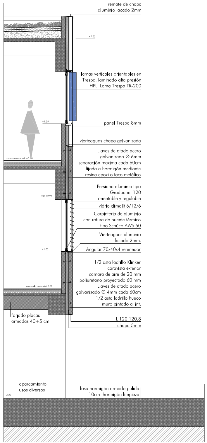
DETALLE FACHADA
